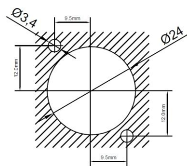
开孔尺寸图
